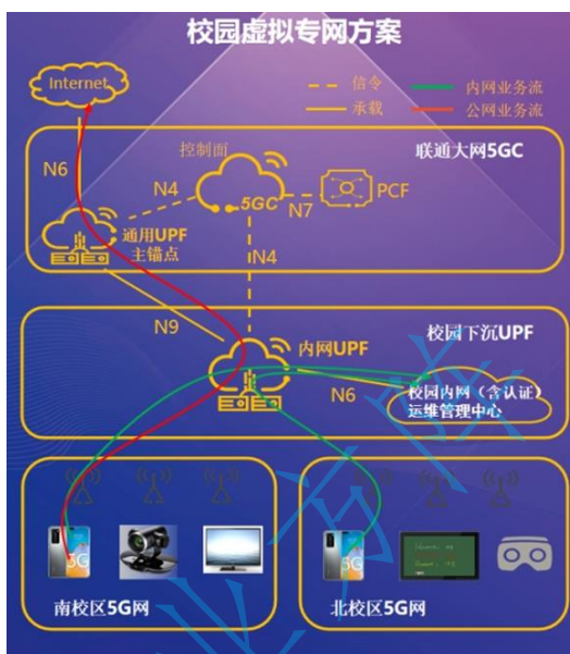
图 31 校园 5G 虚拟专网方案
